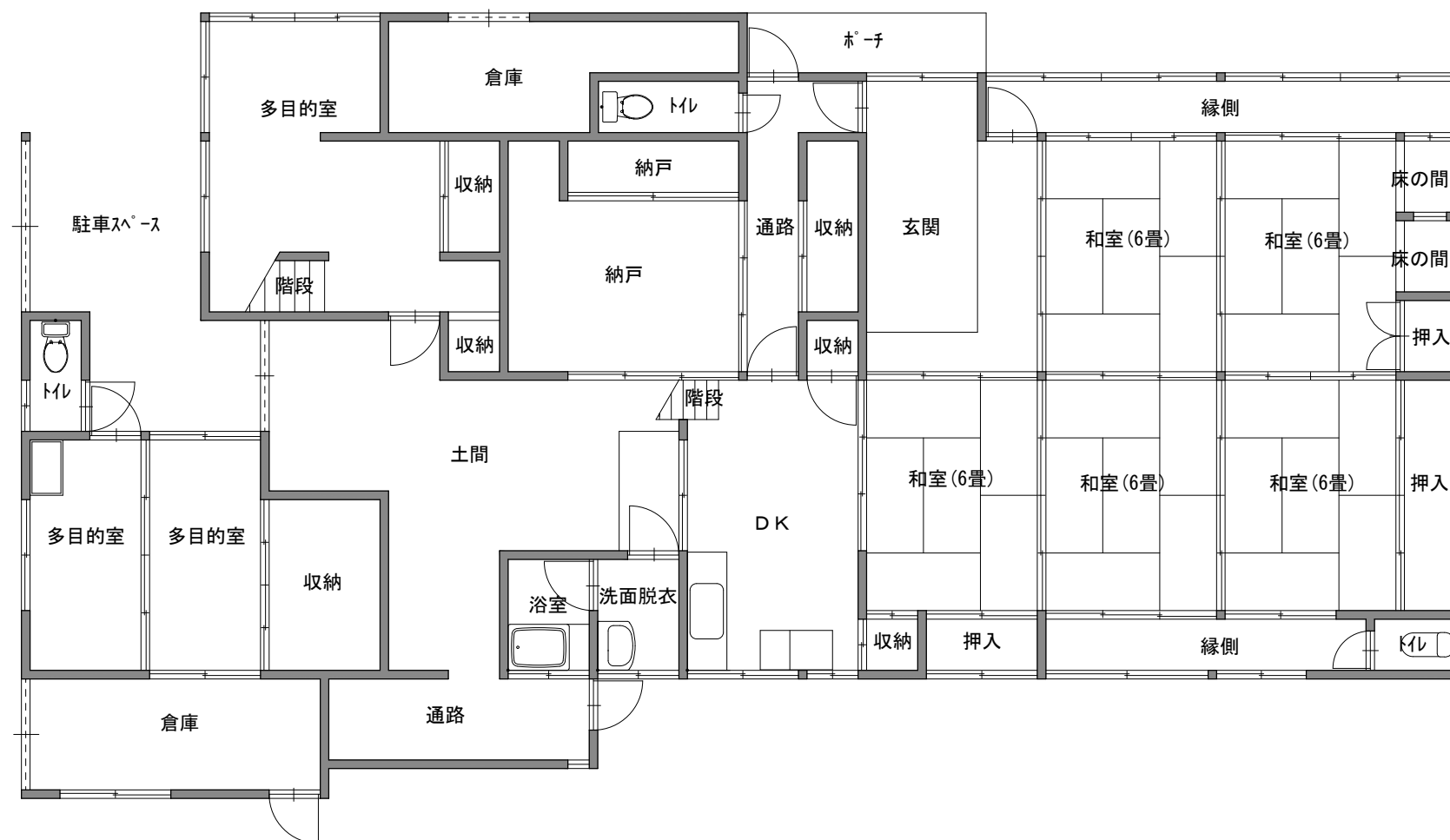
1 階 平 面 図
